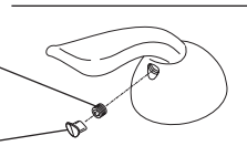
RP40650 Set Screw Tornillo de Ajuste Vis de calage RP51343 Red/Blue Button Botón-Rojo/Azul Bouton-Rouge/Bleu
