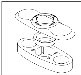
RP101074▲ Escutcheon with Gasket (3 Hole) Chapetón y Empaque (3 agujeros) Boîtier et Joint (3 trous)
